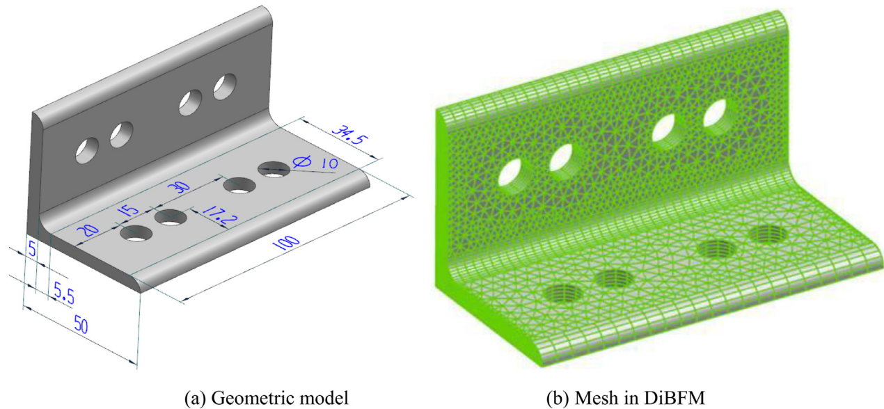
Fig. 26. Angle steel.
